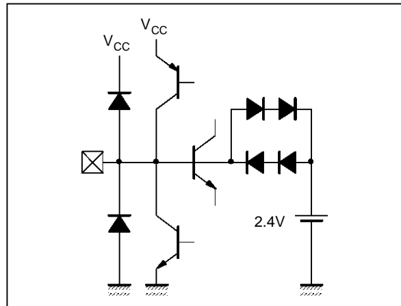
Pin : TRIVADJ
