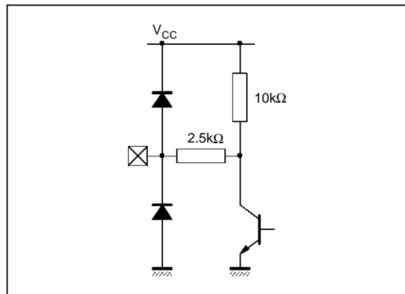
Pin : VSPLP
