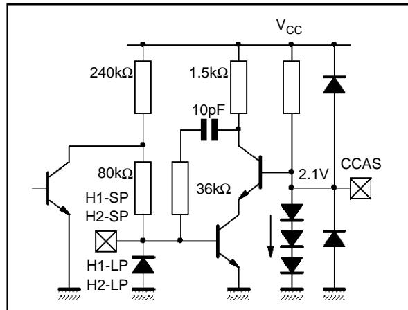
Pin : VSPLP
