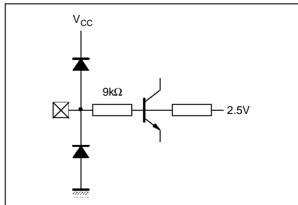
Pin : TRIVADJ
